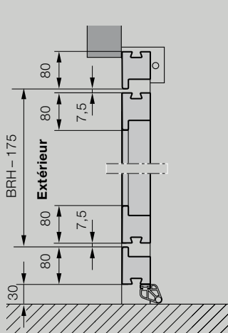
Porte basculante ET 500 avec portillon incorporé
